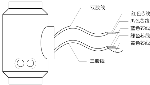
图 4.3.1 信号线处理
